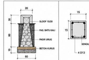
DETAIL PONDASI SKALA 1 : 20
